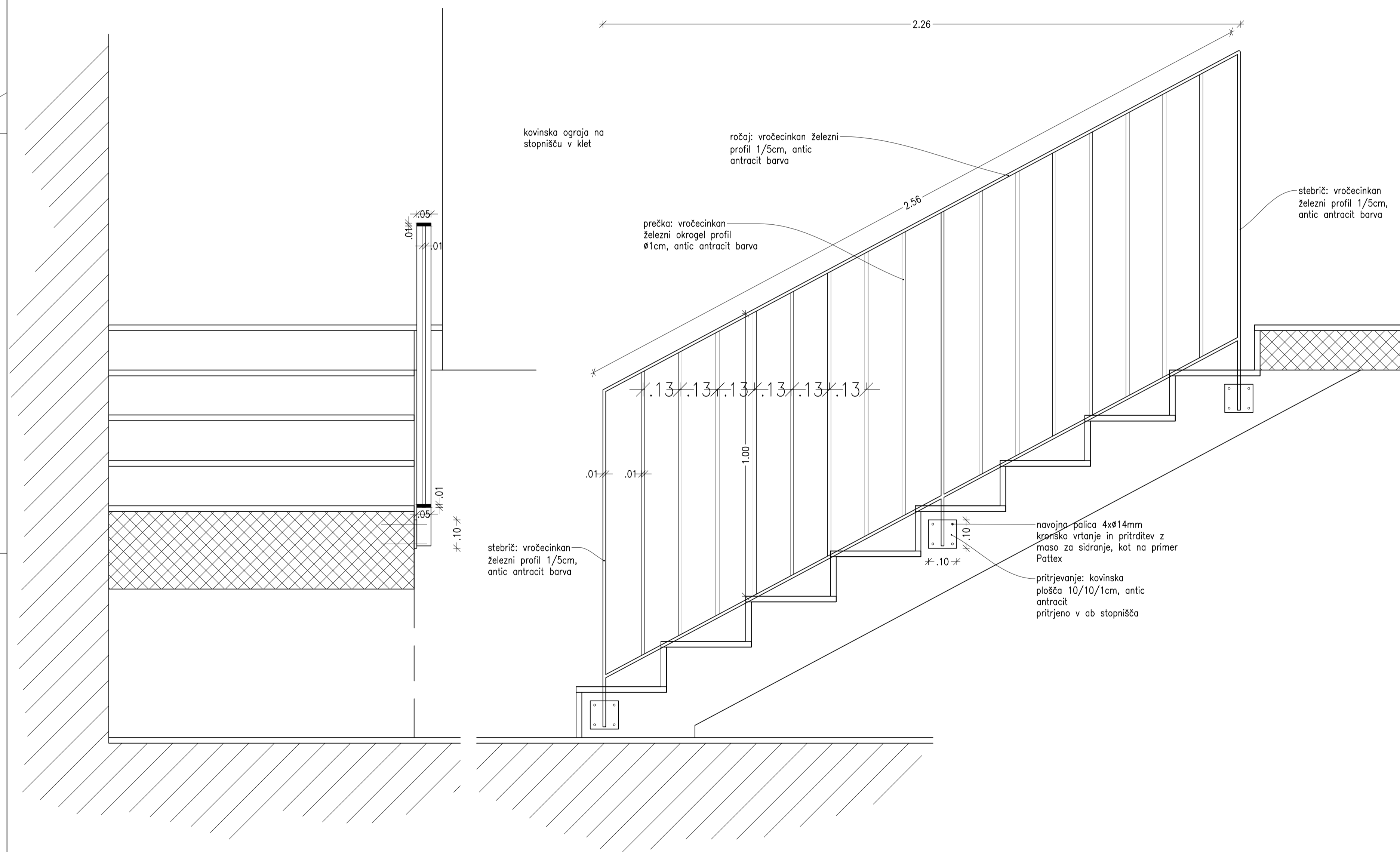
DETALJ KOVINSKE OGRAJE NA STOPNIŠČU V SANITARJE PRITLIČJE/KLET
