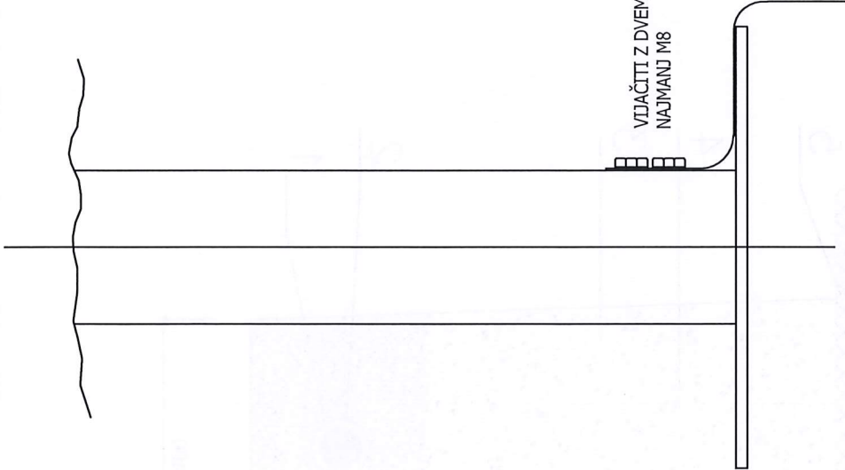
PROTIKOROZIJSKO ZAŠČITEN VALJANEC DO GLOBINE 30cm POD POVRŠINO TAL
